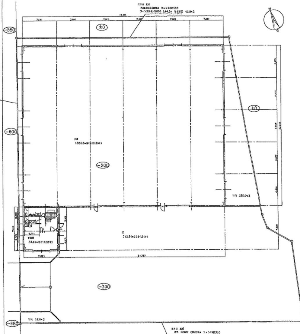
配置図・1階平面図 S=1:300
