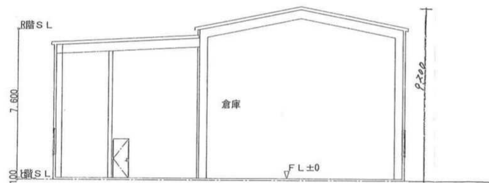
断面図 S:1/150
