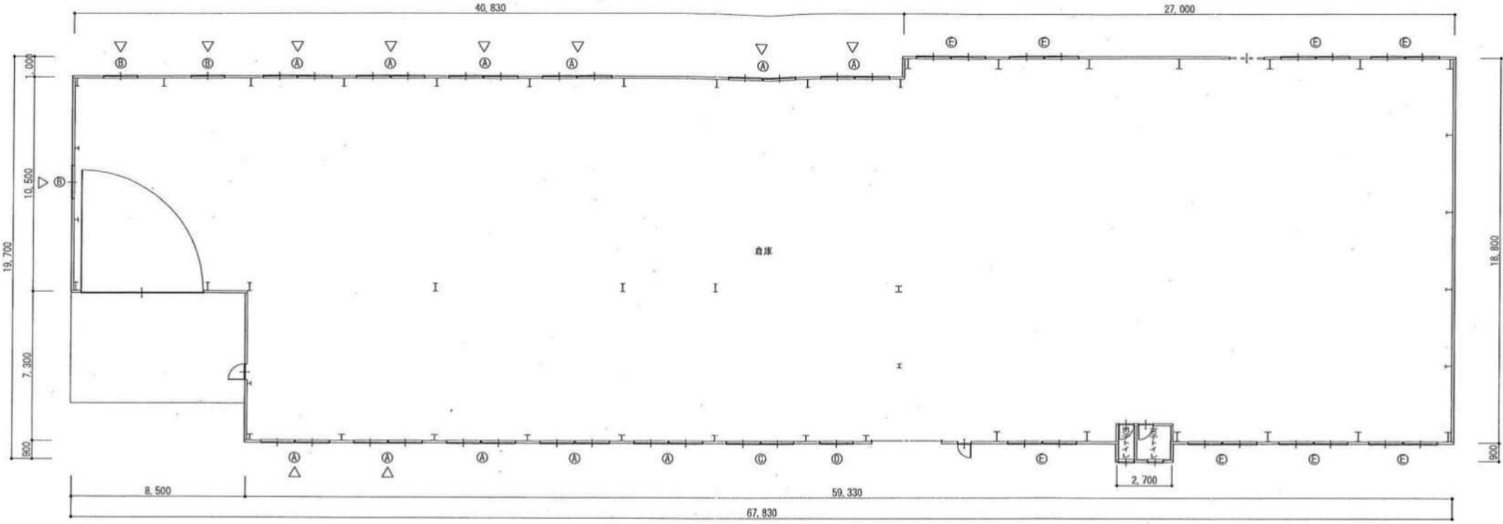
平面図 S:1/200
