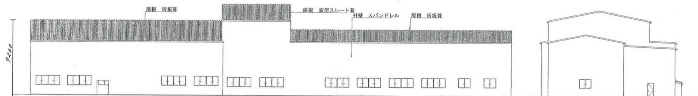
北側 立面図 S:1/250
