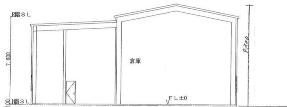
断面図 S:1/150
