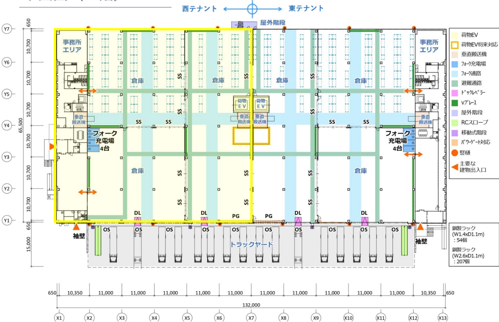
平面図（1階）
