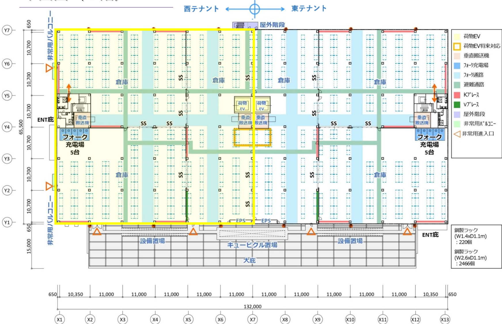
平面図（2階）
