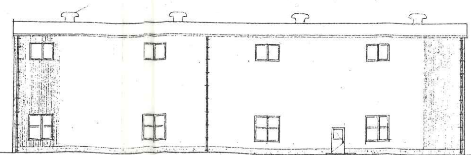
西立面図 S=1:200
